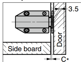
Overlay Door
