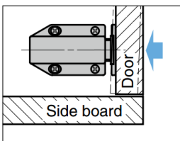
Inset Door
